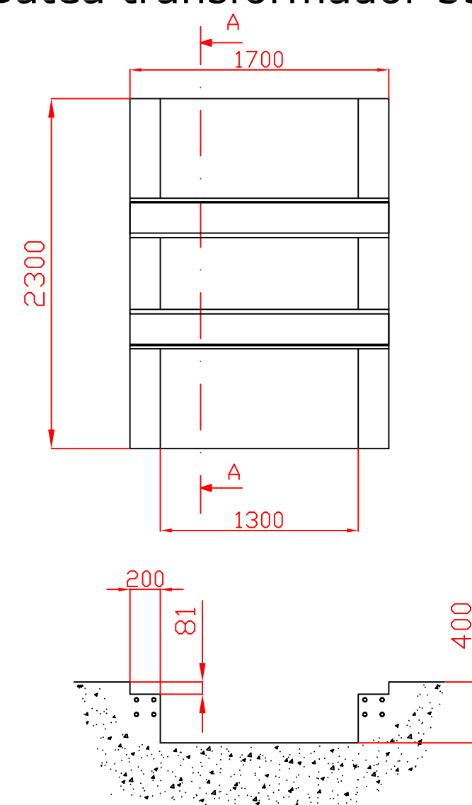
Batea transformador 33/0,4 kV
