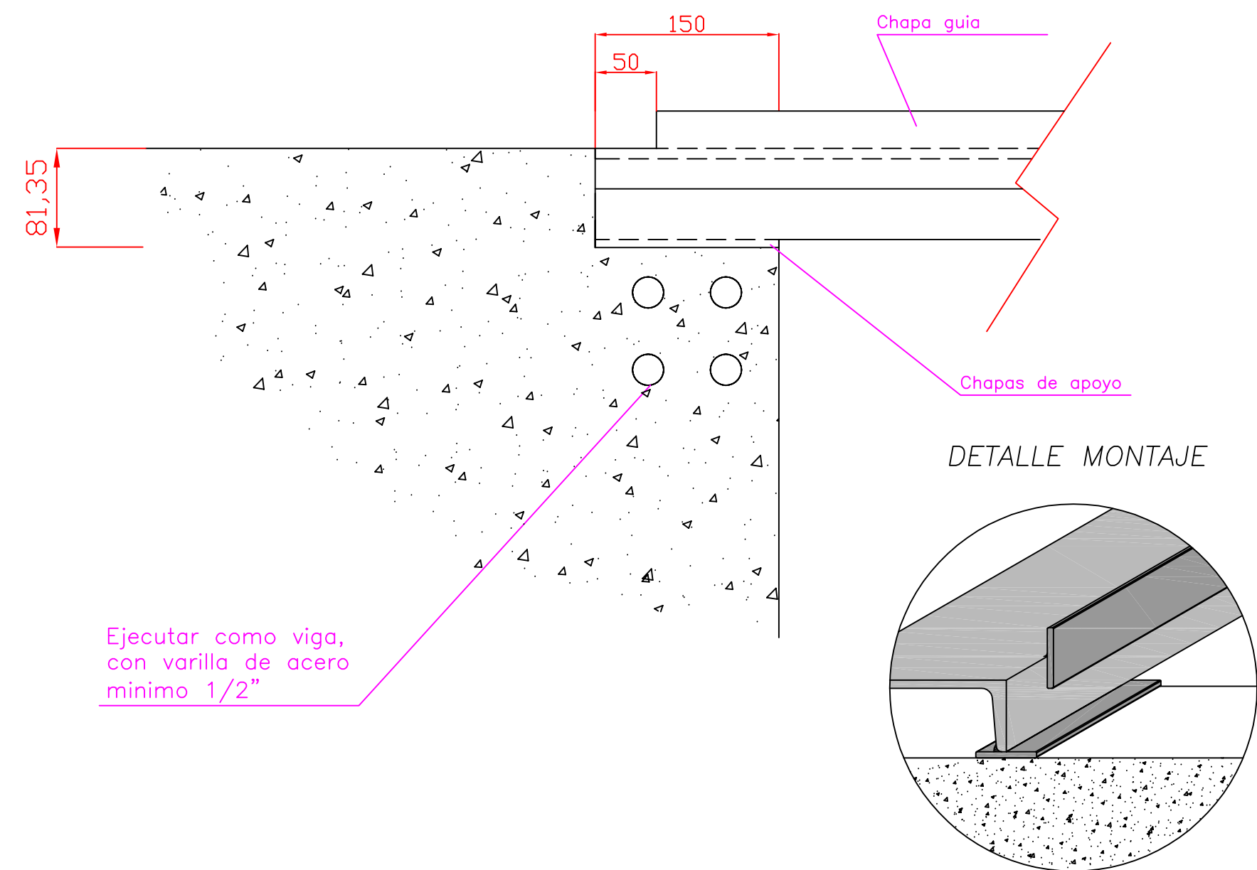
Batea transformador 13,2/0,4 kV
