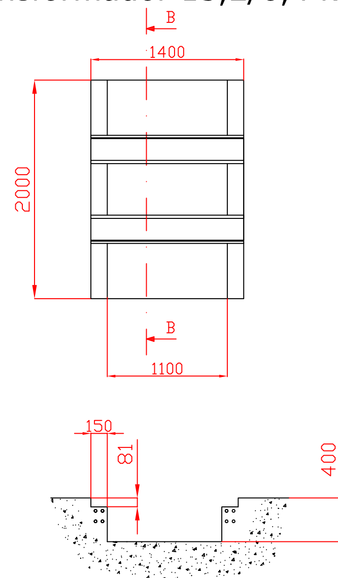
Batea transformador 13,2/0,4 kV
