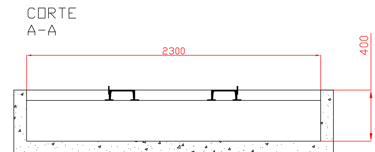
Batea transformador 33/0,4 kV
